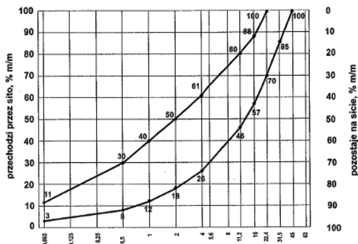
Rys. 2. Krzywe graniczne uziarnienia dla kruszywa 0/31,5.
